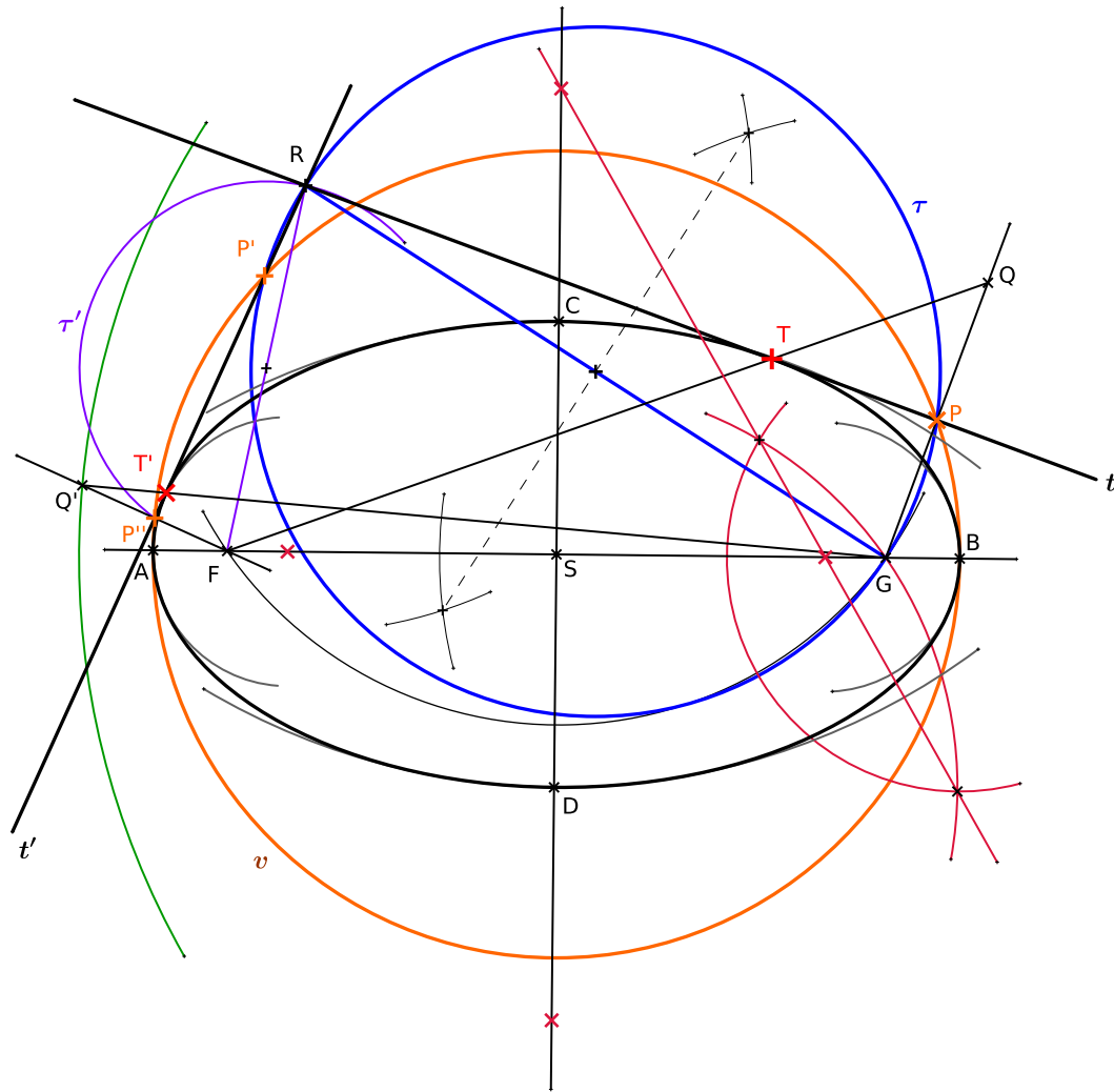
Př. 4 : Sestrojte tečny z vnějšího bodu R k elipse \varepsilon dané osovým křížem AB, CD .
