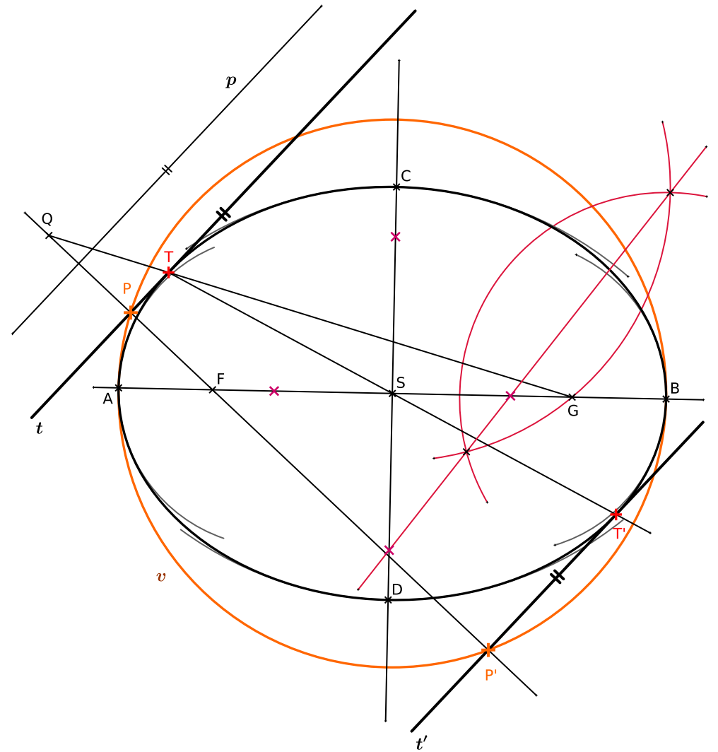
Př. 5 : Sestrojte tečny rovnoběžné s danou přímkou p k elipse \varepsilon(A, F, S) .
