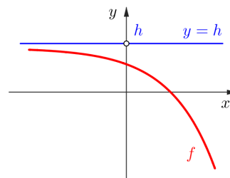
Shora ohraničená funkce
